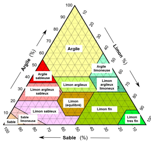
Schéma classique de la texture et de la porosité des sols leurs galeries sont très connectées.
